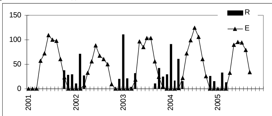
Рис. 2. Рассчитанное питание ПВ (R) и фактическая эвапотранспирация (E) для периода 2001-2005 гг., модель WATBUG (ДПВ = 200 мм)
