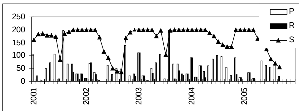
Рис. 1. Месячные осадки (P), питание ПВ (R) и фактический запас влаги в почве (S) в мм слоя за 2001-2005 гг., модель WATBUG (ДПВ = 200 мм)
